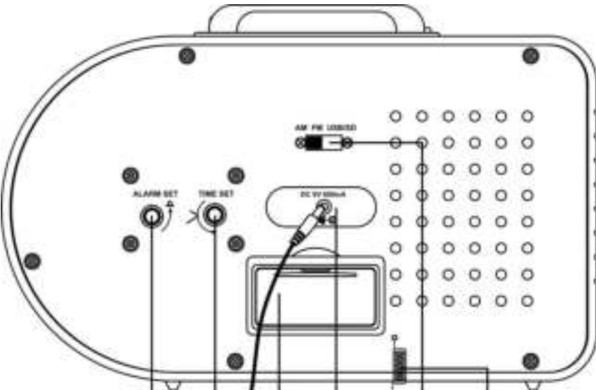
ALARMEINSTELLUNGSKNOPF ZEITEINSTELLUNGSKNOPF NOTSTROMVERSORGUNG DURCH BATTERIEN NETZADAPTER ADAPTERBUCHSE AM FM USB/SD-FREQUENZSCHALTER UKW-DRAHTANTENNE
