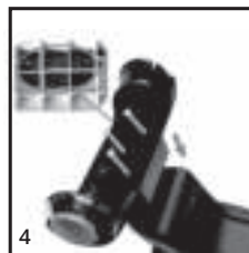
Abbildung 4: Die Hinterradbaugruppe (Teil 5) in die Karosserie (Teil 1) montieren und die Schnalle schließen, dann die drei Schrauben (Teil 3) in die Brücke des Hinterrads (Teil 5) montieren und festziehen.
