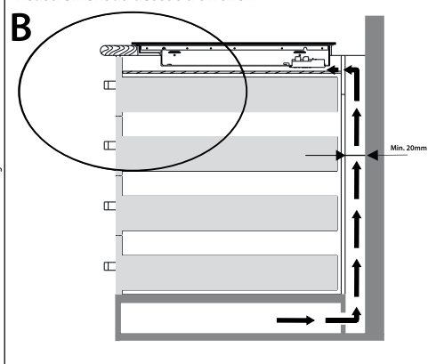
Encastrement au dessus d'un tiroir - B
