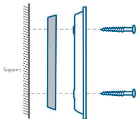
Montage de Cale Montage de mural
