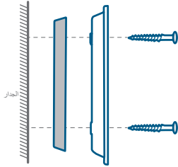
التركيب الإسفين الكتيفة بإسفين متصاعد بمقدار 15 درجة
