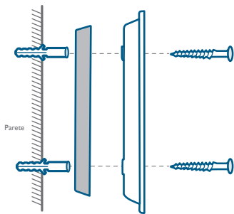
DELLA TELECAMERA PER INTERNI Cuneo
