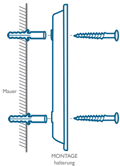
Ohne 15°-Montagekeil
