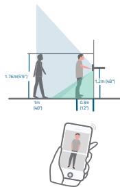
Sem a Cunha de instalação de 15°
