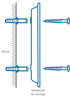
Sin cuña de montaje de 15°
