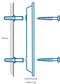
Ohne 15°-Montagekeil
