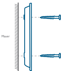
MONTAGE halterung
