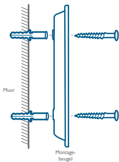
Zonder montagewig van 15°
