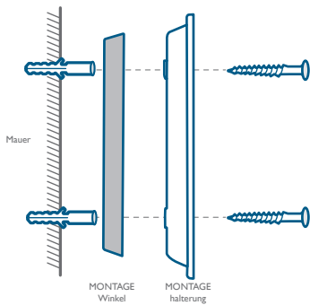
Mit 15°-Montagekeil
