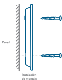
Sin cuña de montaje de 15°
