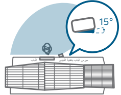
بإسفين تركيب 15°
