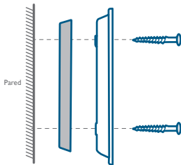
Instalación Cuña Instalación de montaje
