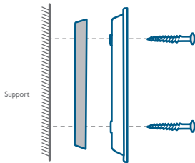
Montage de Cale Montage de mural
