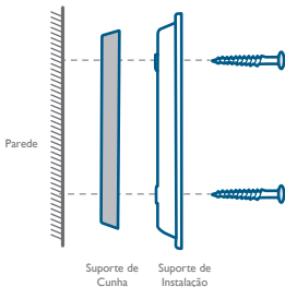
Com a cunha de instalação de 15°
