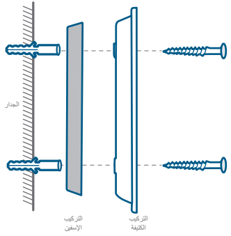
بإسفين متصاعد بمقدار 15 درجة
