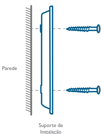
Sem a cunha de instalação de 15°
