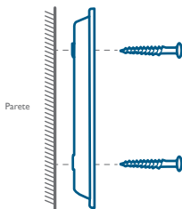
DELLA TELECAMERA PER INTERNI Staffa
