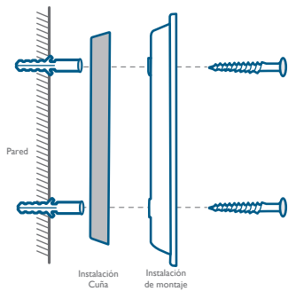
Con cuña de montaje de 15°
