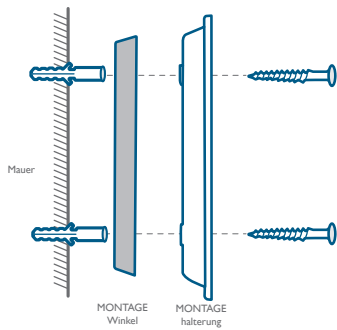
Mit 15°-Montagekeil
