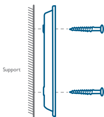
Montage de mural
