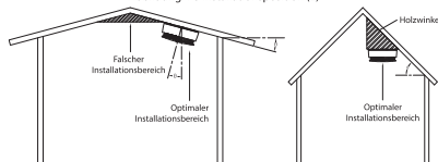
Abbildung 4-3 Installationsposition (2)
