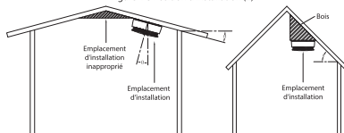
Figure 4-3 Position d'installation (2)
