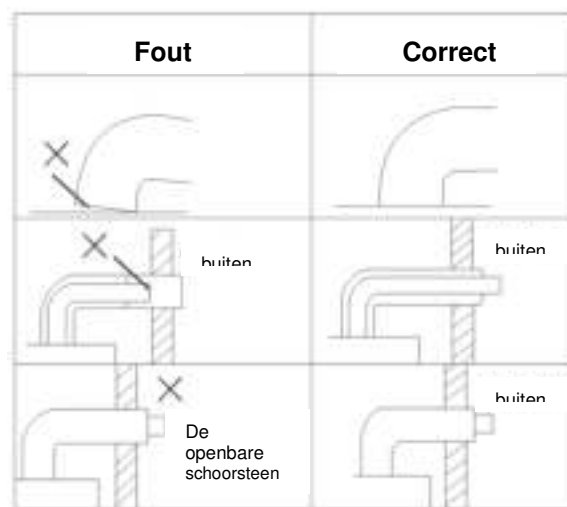
Installatie van de uitlaatpijp
