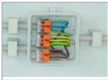
Aansluiting van fijnaderige geleiders in lasdozen
